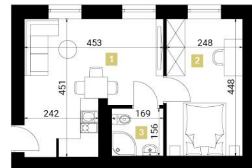
Rzut lokalu
